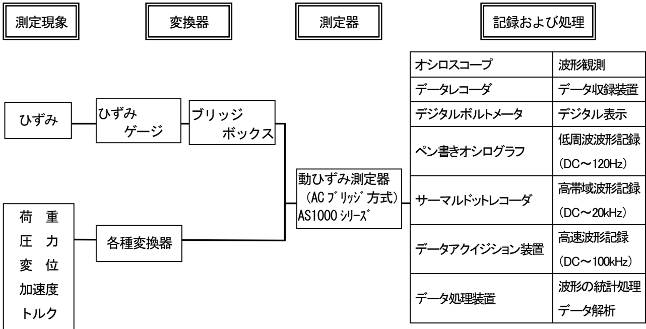
図1-1 計測ブロック図
