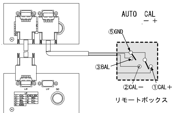
図3-11 リモートボックスの概略図
