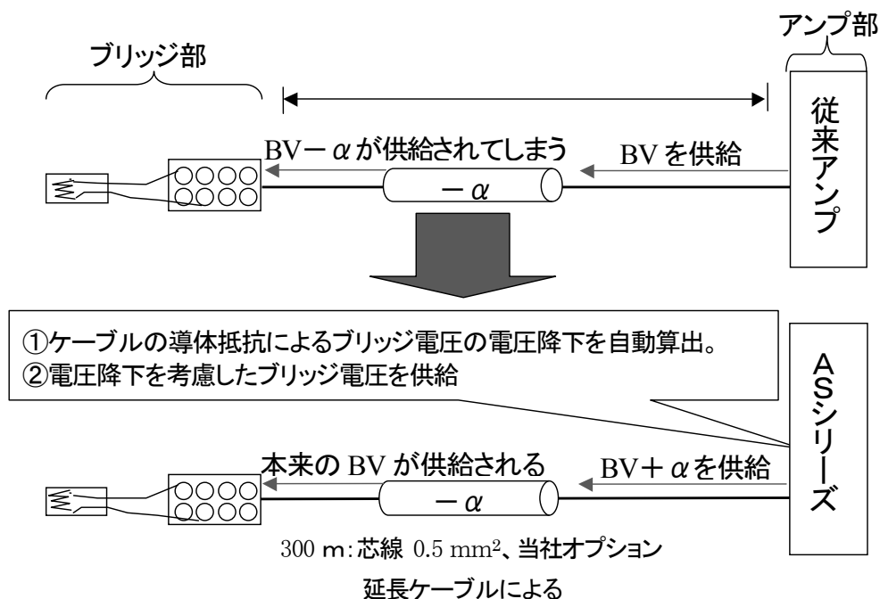
図3-5 線長補正機能の概略図
