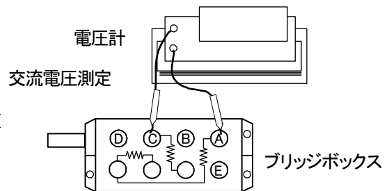
図 4-8 ブリッジ部の電圧測定
