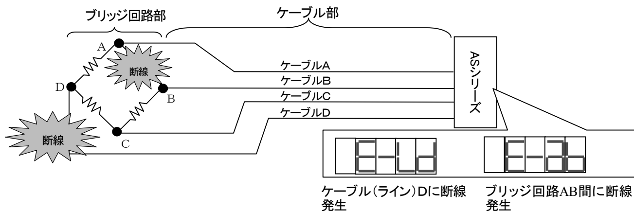
図3-3 断線チェック概略図
