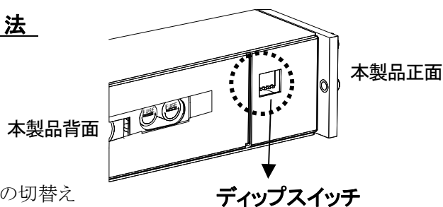
図3-6 ディップスイッチの位置
