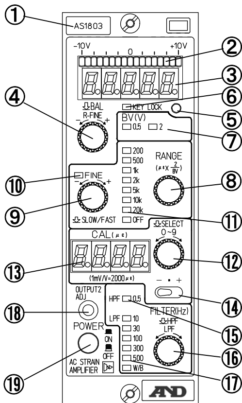
図 2-1 : AS 本体正面
