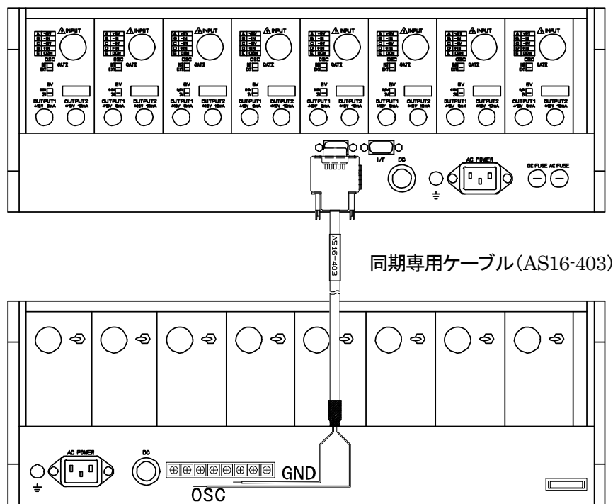
図3-12 旧ケースと新ケースの接続
