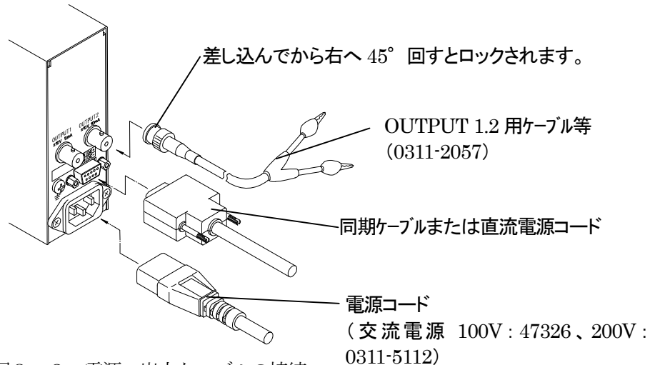
図3-2 電源、出力ケーブルの接続
