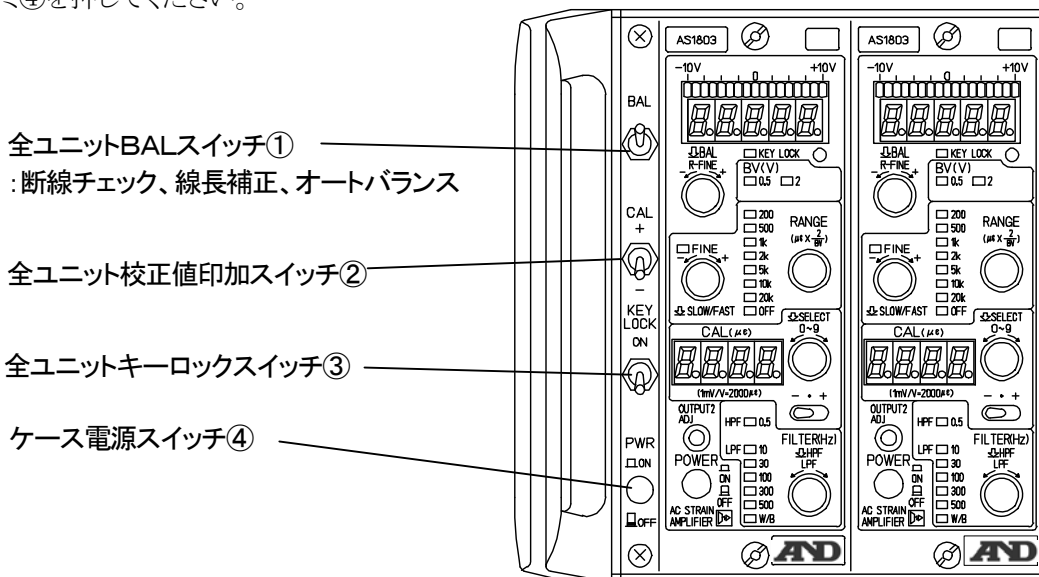
図3-10 ケース正面図
