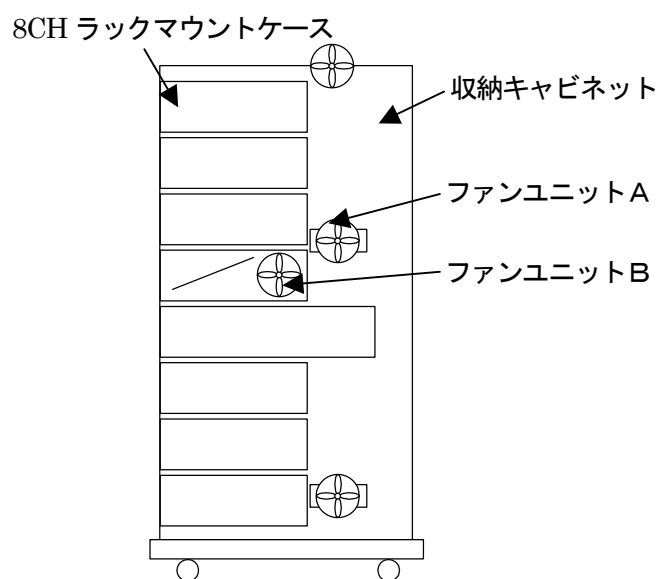
図3-14 ファンの配置箇所
