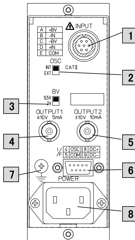
図 2-2 : AS 本体背面
