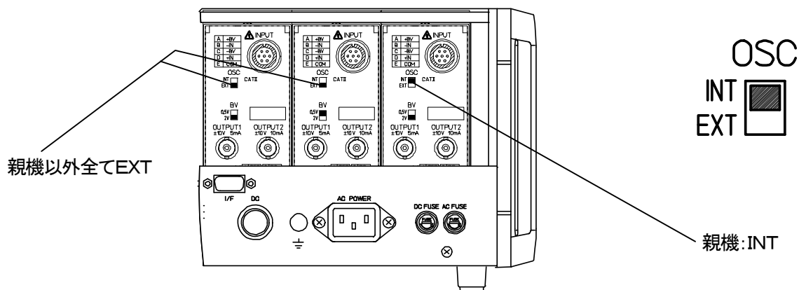
図3-8 ケース背面図
