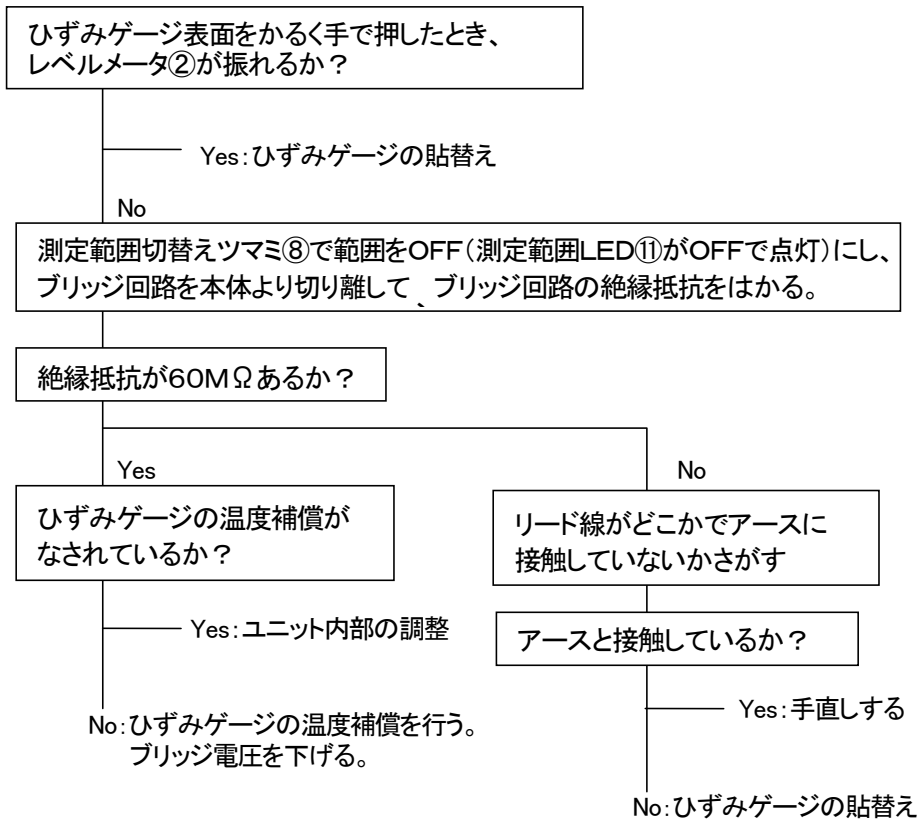
図7-1 確認項目チャート図(2)
