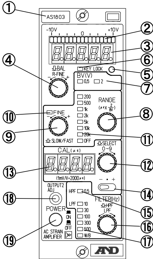
図2-1：AS本体前面
