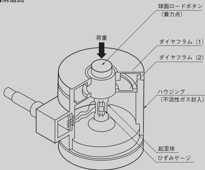
■構造図
