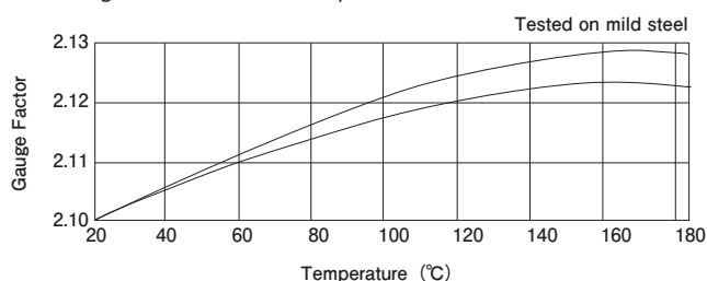
Fig 2 温度によるゲージ率の変化 Gauge Factor variation with temperature
