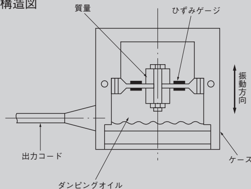
■構造図
